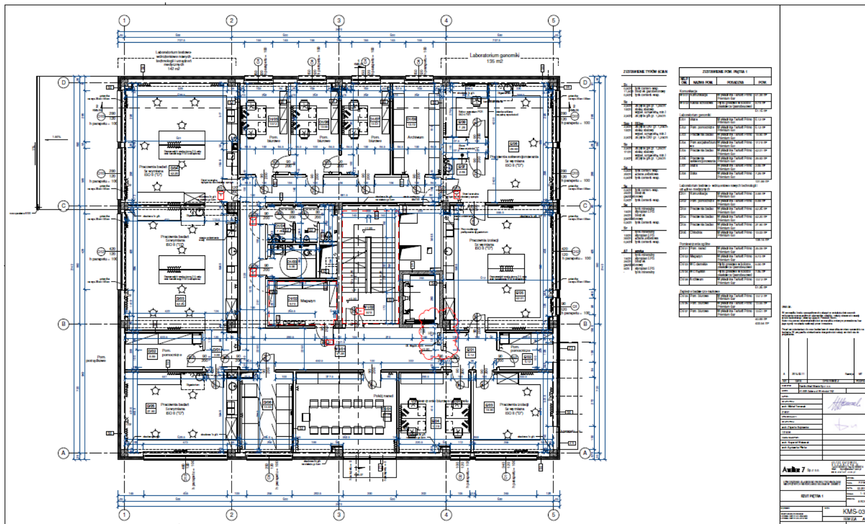
Rzut kondygnacji 1
