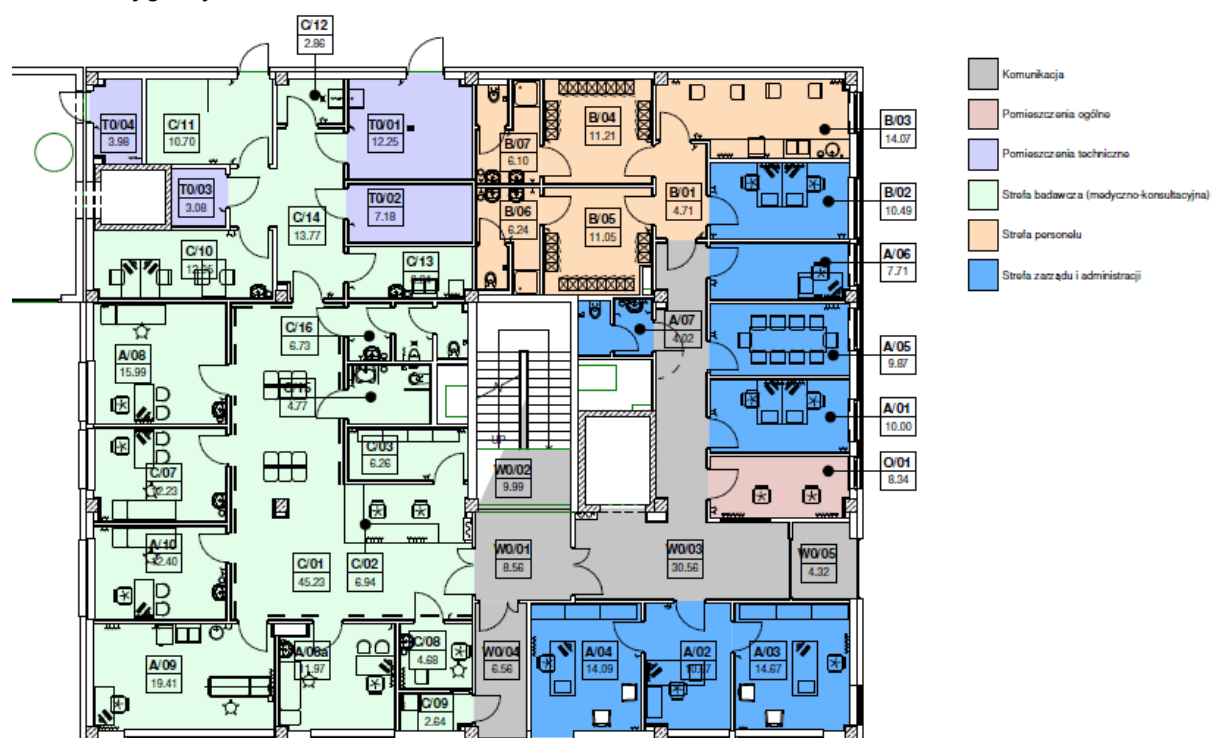
Rzut kondygnacji 0
